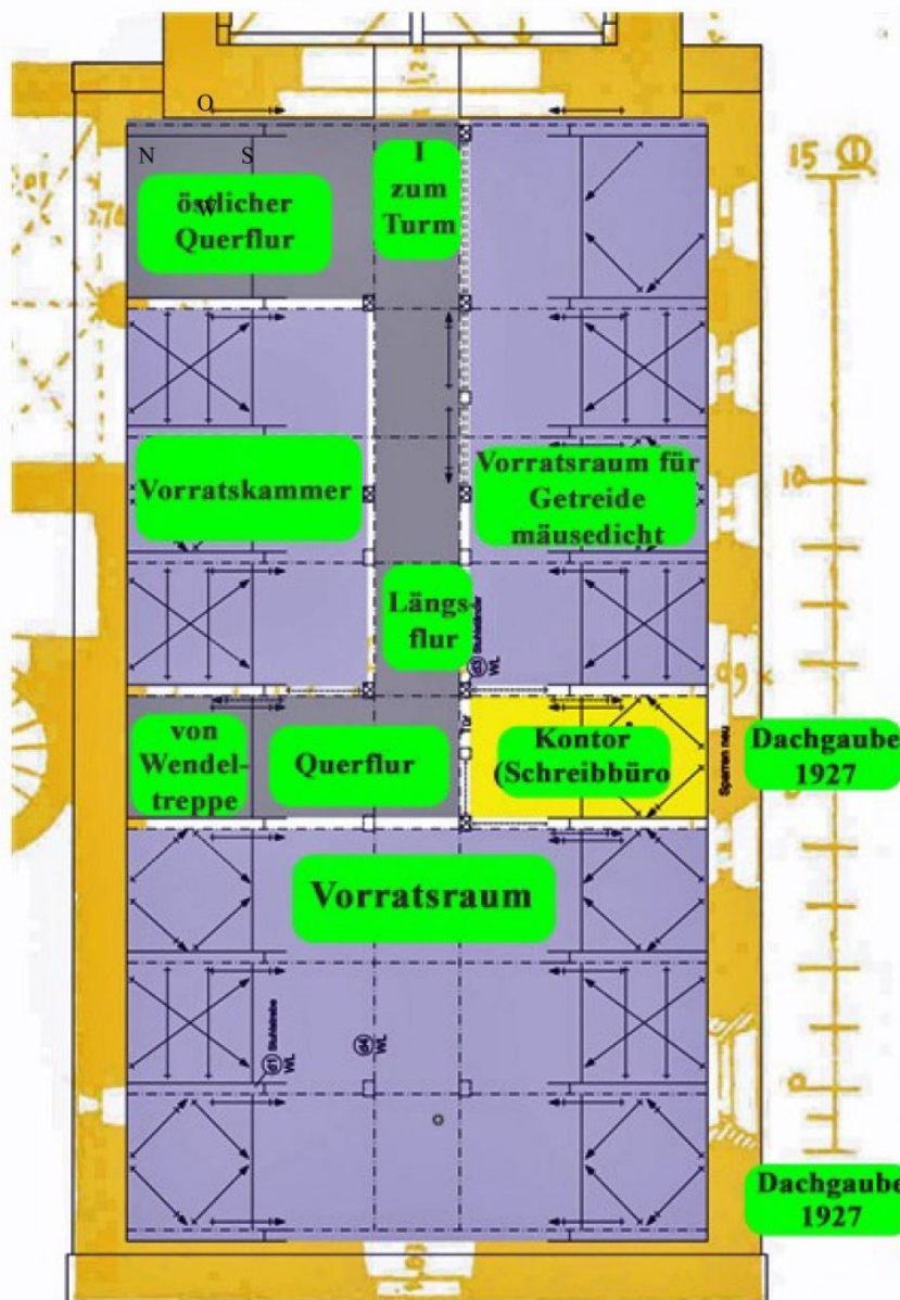
Langhausdachwerk mit Raumaufteilung
